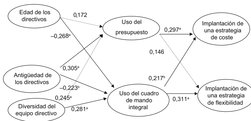
Figura 2. Modelo analizado con la técnica de mínimos cuadrados parciales (PLS).
