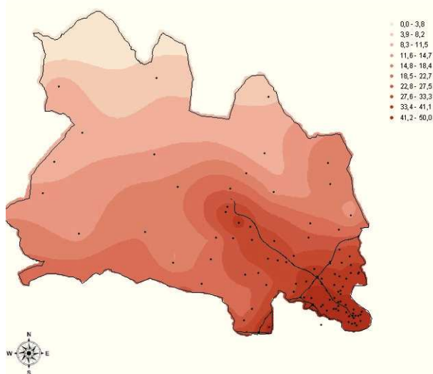
Figura 1. Concentraciones de dióxido de nitrógeno (medido en \mu\text{g}/\text{m}^3 ) estimados a partir de las mediciones del enrejado de la campaña de abril de 2004. Área de estudio de Valencia.
